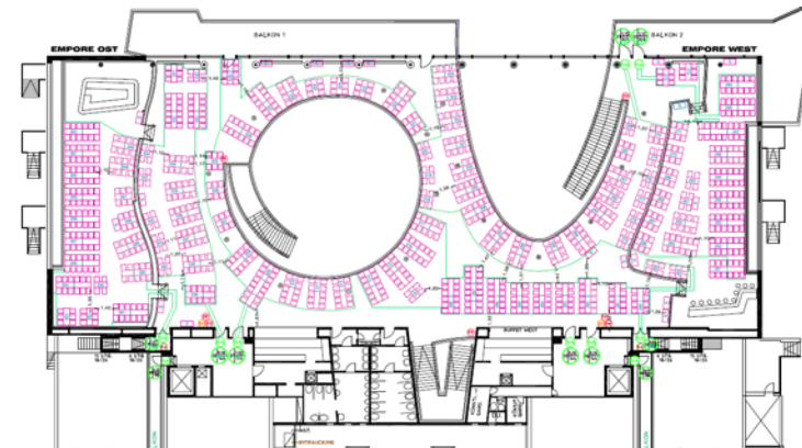
Grundriss OG Plan 93 – Floor plan upper floor # 93
